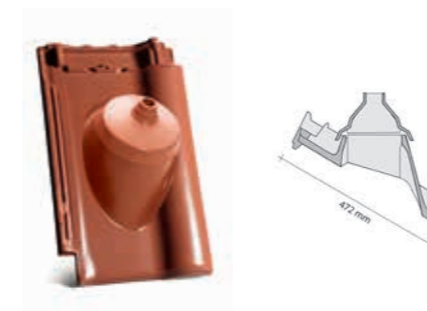
anténní komplet: prostupová taška s pryžovým nástavcem - hmotnost tašky cca: 4,1 kg - pryžový nástavec cca: 0,1 kg - hmotnost 1 ks cca: 4,2 kg
