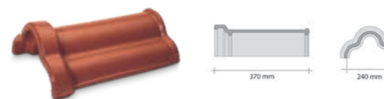
hřebenáč drážkový s přichytkou - potřeba na 1 bm cca: 3,0 ks/bm - hmotnost 1 ks cca: 3,6 kg/ks - krycí šířka cca: 20,5 cm
