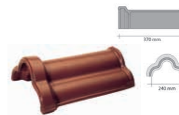
hřebenač drážkový s příchtykou - potřeba na 1 bm 3,0 ks/bm - hmotnost 1 ks cca: 3,6 kg/ks - krycí šířka cca: 20,5 cm
