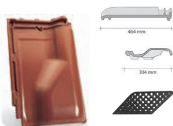
větrací taška - větrací průměr cca: 23 cm 2 - hmotnost 1 ks cca: 3,9 kg Součástí tašky je mřížka do otvoru proti škůdcům.
