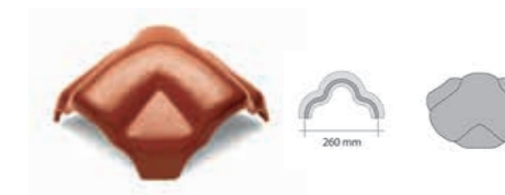
rozbočovací hřebenáč univerzální Y, univerzální, dostupný je i ve tvaru X nebo T - hmotnost 1 ks cca: 4,8 kg
